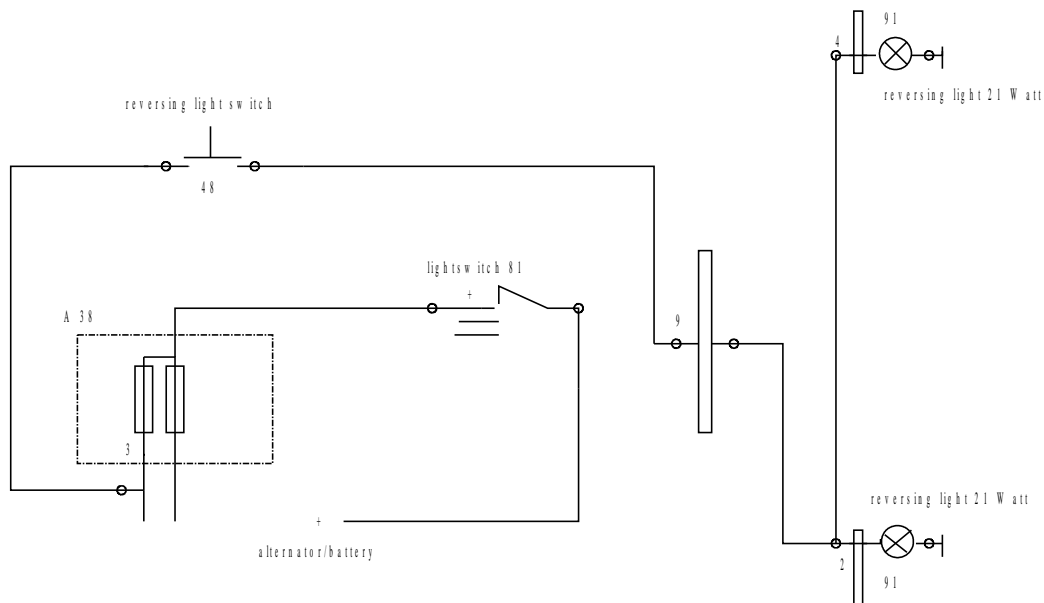
Fig. 1 Voorbeeld van een deelschema van het achteruitrijd-verlichtingscircuit
